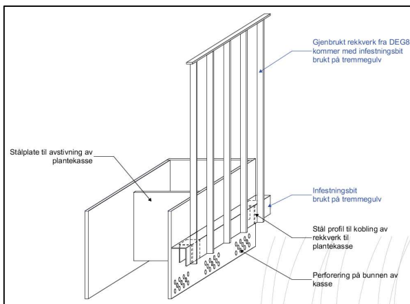
Detalj av innfesting til plantekasse. MAD arkitekter.
