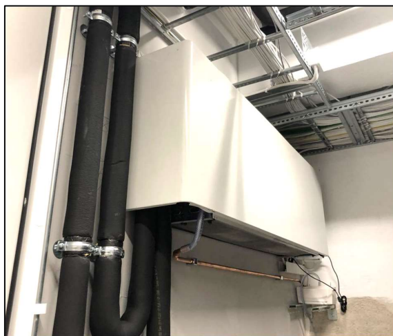
Ombrukt viftekonvektor montert i datarom i kjeller. Foto: Rune Andersen
