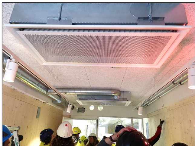
Bafler ferdig montert i prøverom i KA13. Foto: Christoffer Siopan Engtrø
