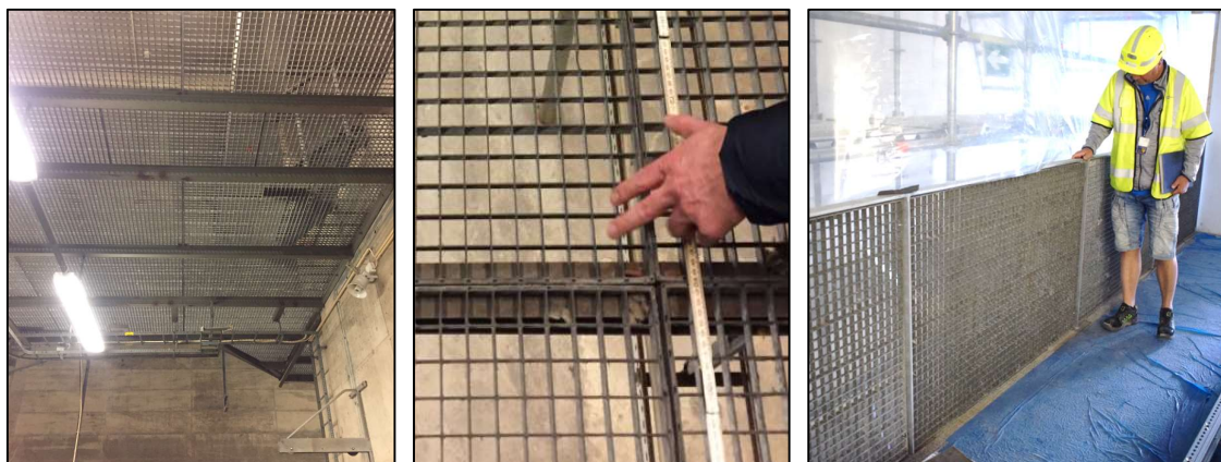
1-2: Gitterrister som gulv i teknisk rom på Tøyenbadet, og oppmåling av disse under befaring. Foto: Catriona Shine.
